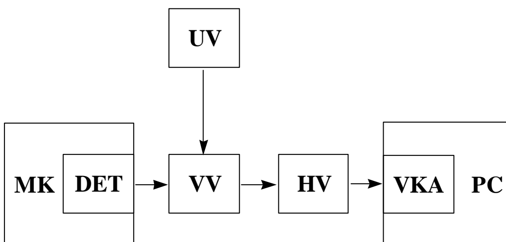
Abb. 1: Blockschaltbild des Messplatzes.
