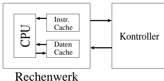
Abbildung 5.1.2: Harvard-Architektur in modernen Prozessoren
