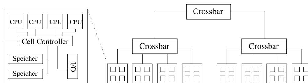
Abbildung 5.2.3: HP 9000 Superdome
