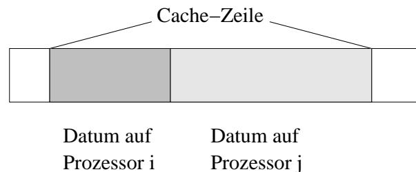
Abbildung 8.1.1: False-Sharing: Daten auf unterschiedlichen Prozessoren benutzen die gleiche Cache-Zeile
