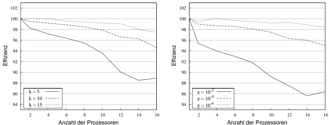
Abbildung 6.5.2: Parallele Effizienz in Abhängigkeit von k (links) bzw. \epsilon (rechts)
