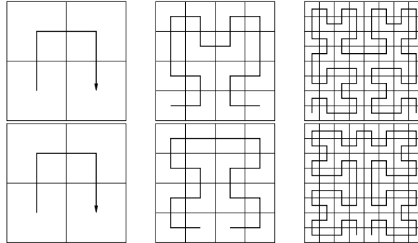
Abbildung 4.2.4: Hilbert-Kurve (oben) und Moore-Kurve (unten)
