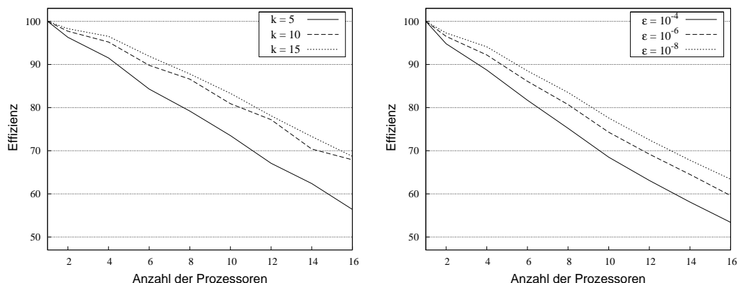
Abbildung 6.6.3: Parallele Effizienz in Abhängigkeit von k (links) bzw. \epsilon (rechts)
