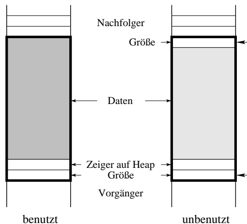
Abbildung 8.4.3: Boundary Tags in Speicherblöcken
