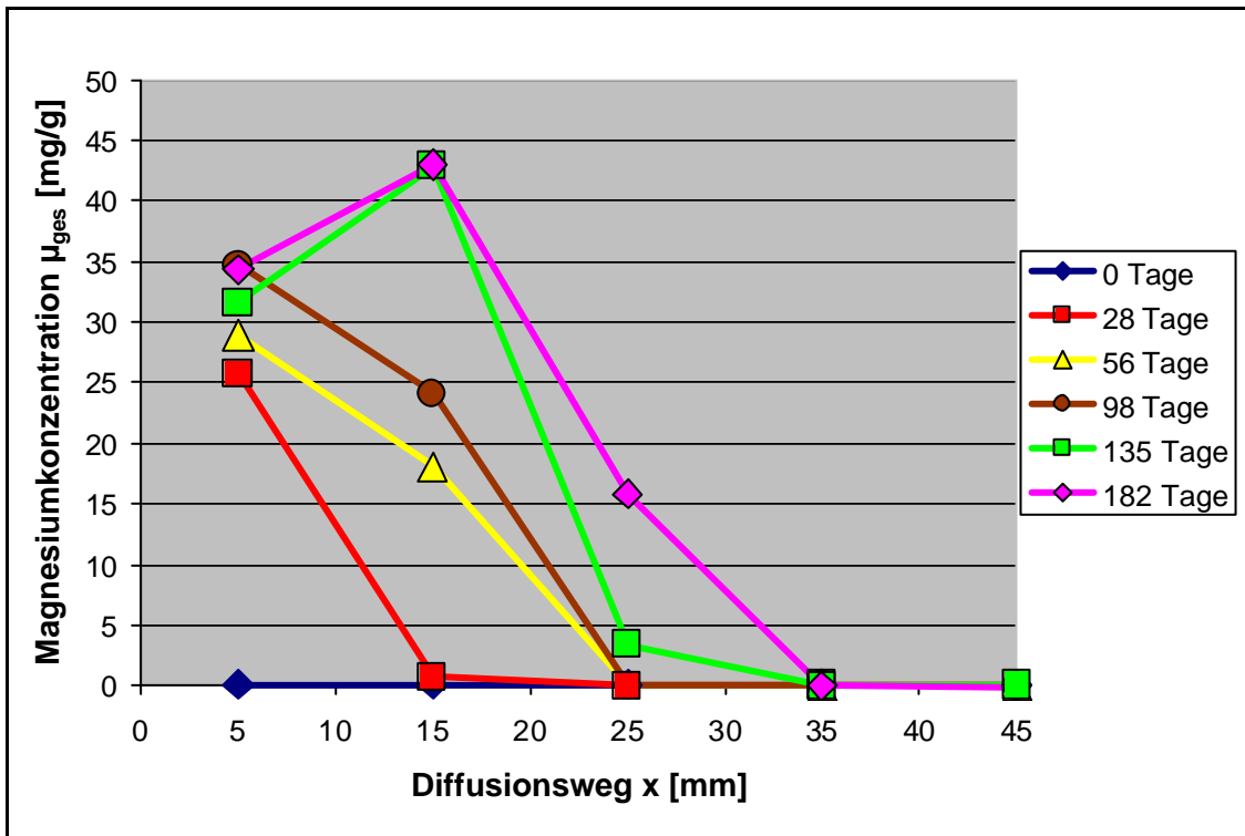
Abb.67: Lagerung in Magnesiumlösung. Magnesiumkonzentration \mu_{ges} in Abhängigkeit vom Diffusionsweg x (Diffusionsprofile) für unterschiedliche Lagerungszeiten. Mg^{2+} -Konzentration 2.000 mg/l. Dichtwandmasse Na-230.
