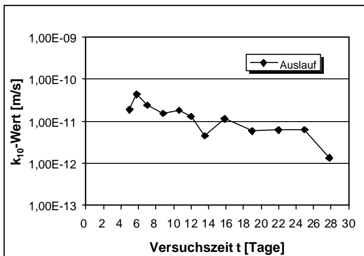
Abb.V.39: Lagerung in Leitungswasser. k_{10} -Wert in Abhängigkeit von der Versuchsdauer nach 98 Tagen Lagerung. Dichtwandmasse Na-540. Messung 1.
