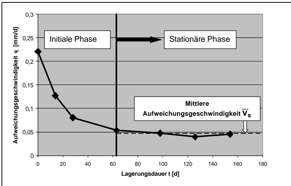
Abb.III.24: Lagerung in kohlensäurehaltigem Wasser. Aufweichungsgeschwindigkeit v_i als Funktion der Lagerungsdauer t . CO_{2(aq)} -Konzentration: 100 mg/l. Dichtwandmasse Na-250.
