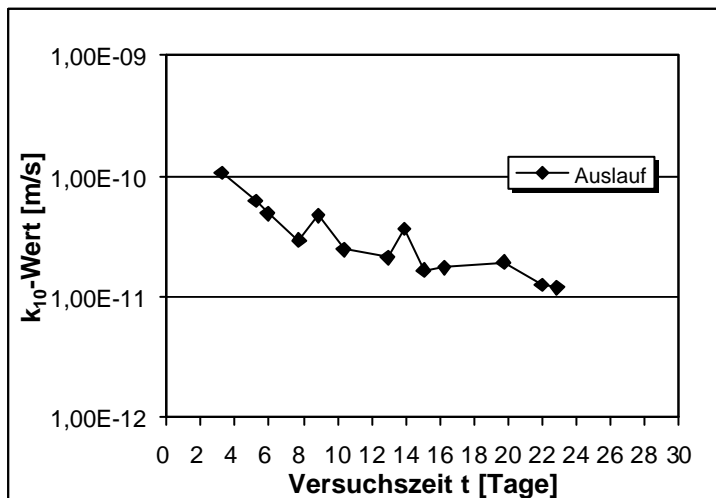
Abb.V.12: Lagerung in Sulfatlösung. k_{10} -Wert in Abhängigkeit von der Versuchsdauer nach 28 Tagen Lagerung. \text{SO}_4^{2-} -Konzentration 7.500 mg/l. Dichtwandmasse Na-230. Messung 2.
