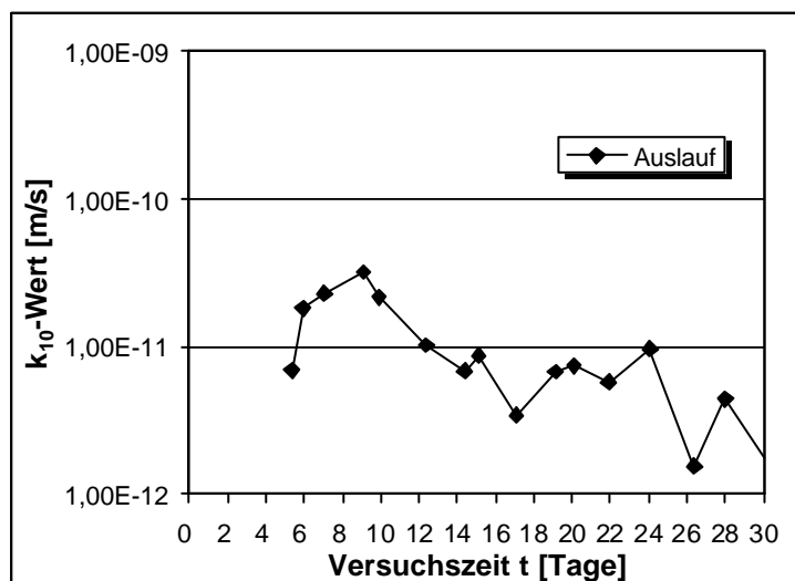
Abb.V.6: Lagerung in Leitungswasser. k_{10} -Wert in Abhängigkeit von der Versuchsdauer nach 56 Tagen Lagerung. Dichtwandmasse Na-230. Messung 2.
