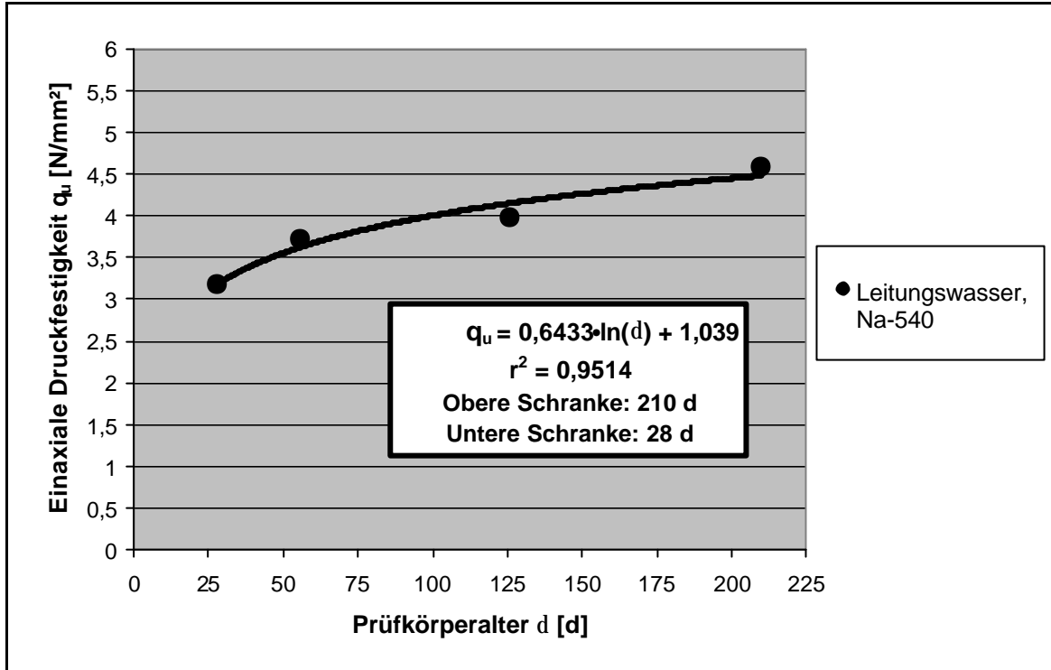
Abb.33: Lagerung in Leitungswasser. Einaxiale Druckfestigkeit q_u als Funktion des Prüfkörperalters \delta . Dichtwandmasse Na-540.
