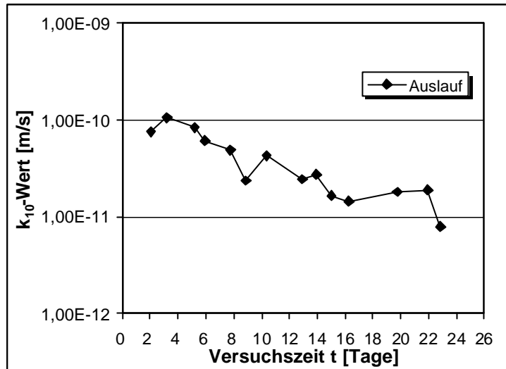
Abb.V.4: Lagerung in Leitungswasser. k_{10} -Wert in Abhängigkeit von der Versuchsdauer nach 28 Tagen Lagerung. Dichtwandmasse Na-230. Messung 3.
