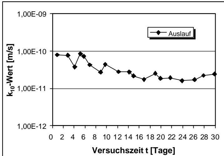
Abb.V.49: Lagerung in Sulfatlösung. k_{10} -Wert in Abhängigkeit von der Versuchsdauer nach 56 Tagen Lagerung. \text{SO}_4^{2-} -Konzentration 15.000 mg/l. Dichtwandmasse Na-540. Messung 4.
