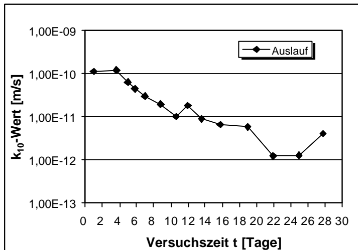
Abb.V.53: Lagerung in Sulfatlösung. k_{10} -Wert als Funktion der Versuchsdauer nach 98 Tagen Lagerung. \text{SO}_4^{2-} -Konzentration 15.000 mg/l. Dichtwandmasse Na-540. Messung 4.
