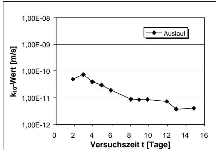
Abb.V.43: Lagerung in Leitungswasser. k_{10} -Wert in Abhängigkeit von der Versuchsdauer nach 182 Tagen Lagerung. Dichtwandmasse Na-540. Messung 3.
