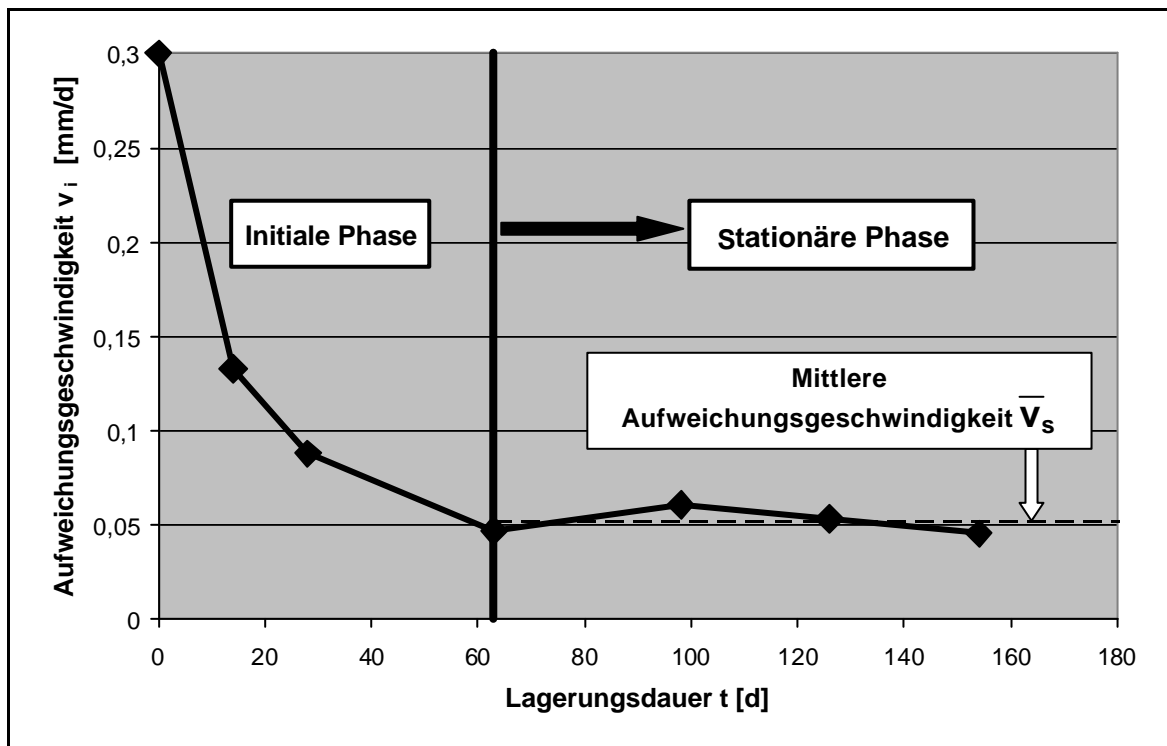
Abb.23: Lagerung in kohlensäurehaltigem Wasser. Aufweichungsgeschwindigkeit v als Funktion der Lagerungsdauer t . \text{CO}_{2(\text{aq})} -Konzentration: 100 mg/l. Dichtwandmasse Na-230.
