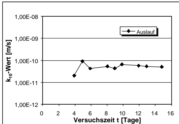
Abb.V.35: Lagerung in Sulfatlösung. k_{10} -Wert in Abhängigkeit von der Versuchsdauer nach 182 Tagen Lagerung. \text{SO}_4^{2-} -Konzentration 15.000 mg/l. Dichtwandmasse Na-230. Messung 2.
