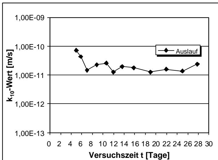
Abb.V.9: Lagerung in Leitungswasser. k_{10} -Wert in Abhängigkeit von der Versuchsdauer nach 98 Tagen Lagerung. Dichtwandmasse Na-230. Messung 2.
