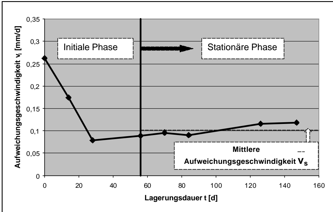
Abb.III.21: Lagerung in Magnesiumlösung. Aufweichungsgeschwindigkeit v_i als Funktion der Lagerungsdauer t . Mg^{2+} -Konzentration: 1.000 mg/l. Dichtwandmasse Na-230.
