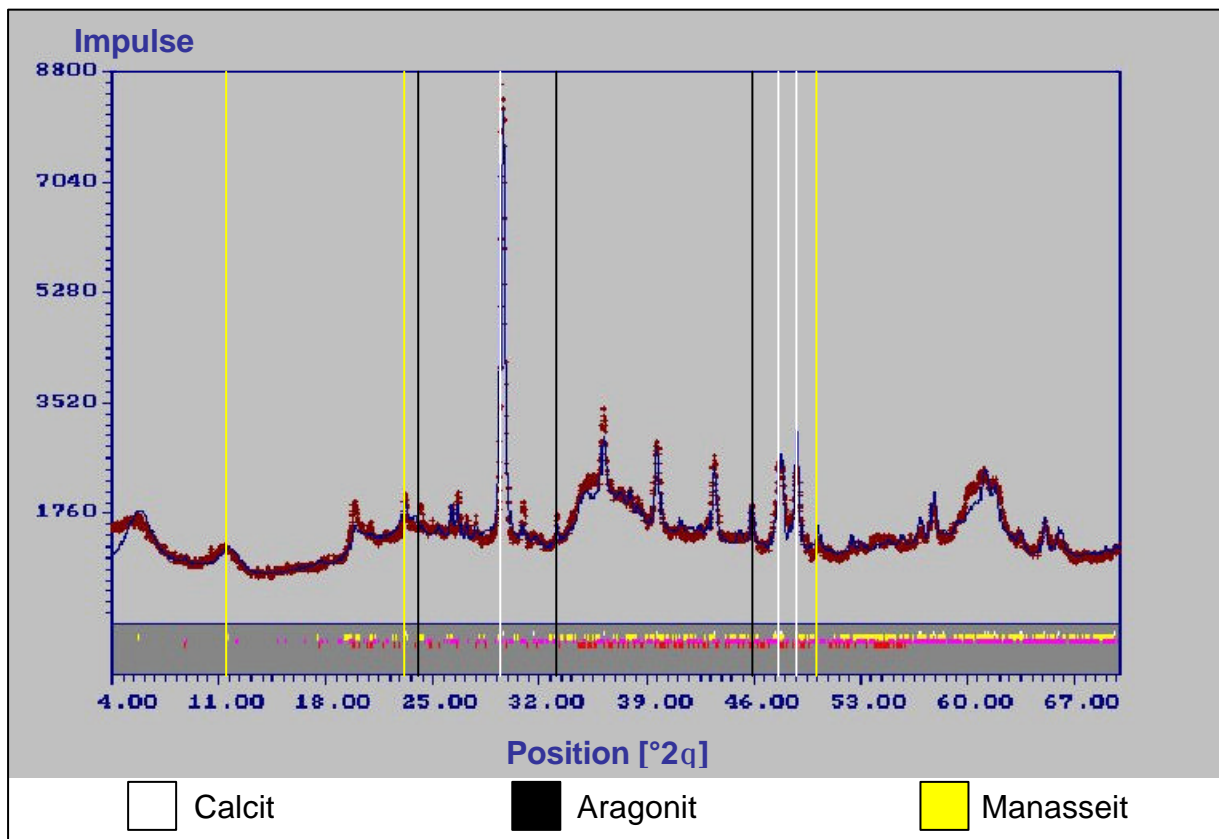
Abb.62: Lagerung in Magnesiumlösung. Röntgendiffraktogramm der Dichtwandmasse Na-230 nach einer Lagerungsdauer von 182 Tagen. Mg^{2+} -Konzentration 2.000 mg/l. Blaue Kurve: Messwerte. Rote Kurve: Berechnete Werte.
