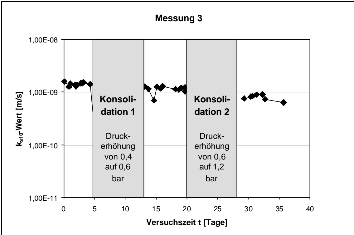
Abb.V.57: Lagerung in Magnesiumlösung. k_{s10} -Wert in Abhängigkeit von der Versuchsdauer t. Dichtwandmasse Na-230. Vor Beginn der Durchströmung 56 Tage Lagerung in einer Magnesiumlösung ( Mg^{2+} -Konzentration: 2.000 mg/l). Mächtigkeit der Aufweichungsschicht 15 mm
