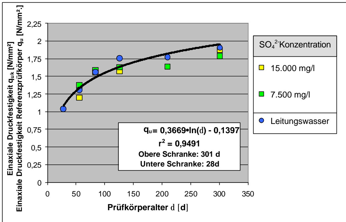
Abb.31: Lagerung in Sulfatlösungen und Leitungswasser. Einaxiale Druckfestigkeit der in Sulfatlösung gelagerten Prüfkörper q_{uk} und der Referenzprüfkörper q_u als Funktion des Prüfkörperalters \delta . Dichtwandmasse Na-230.
