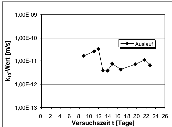
Abb.V.1: Nullprobe. k_{10} -Wert in Abhängigkeit von der Versuchsdauer. Dichtwandmasse Na-230. Messung 1.
