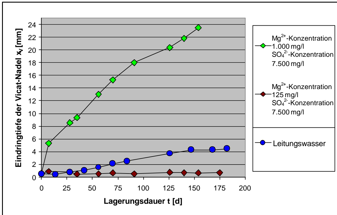
Abb.21: Lagerung in kombinierten Magnesium-/ Sulfatlösungen und Leitungswasser. Eindringtiefe der Vicat-Nadel x_v in Abhängigkeit von der Lagerungsdauer t . Dichtwandmasse Na-230.
