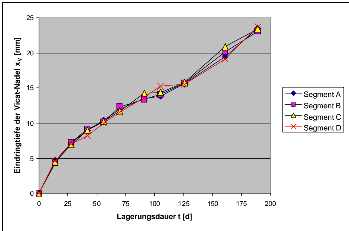
Abb.III.1: Vorversuch. An den Segmenten A bis D gemessene Eindringtiefe der Vicat-Nadel x_v in Abhängigkeit von der Lagerungsdauer t bei einer Magnesiumkonzentration von 1.000 mg/l. Dichtwandmasse Na-230.
