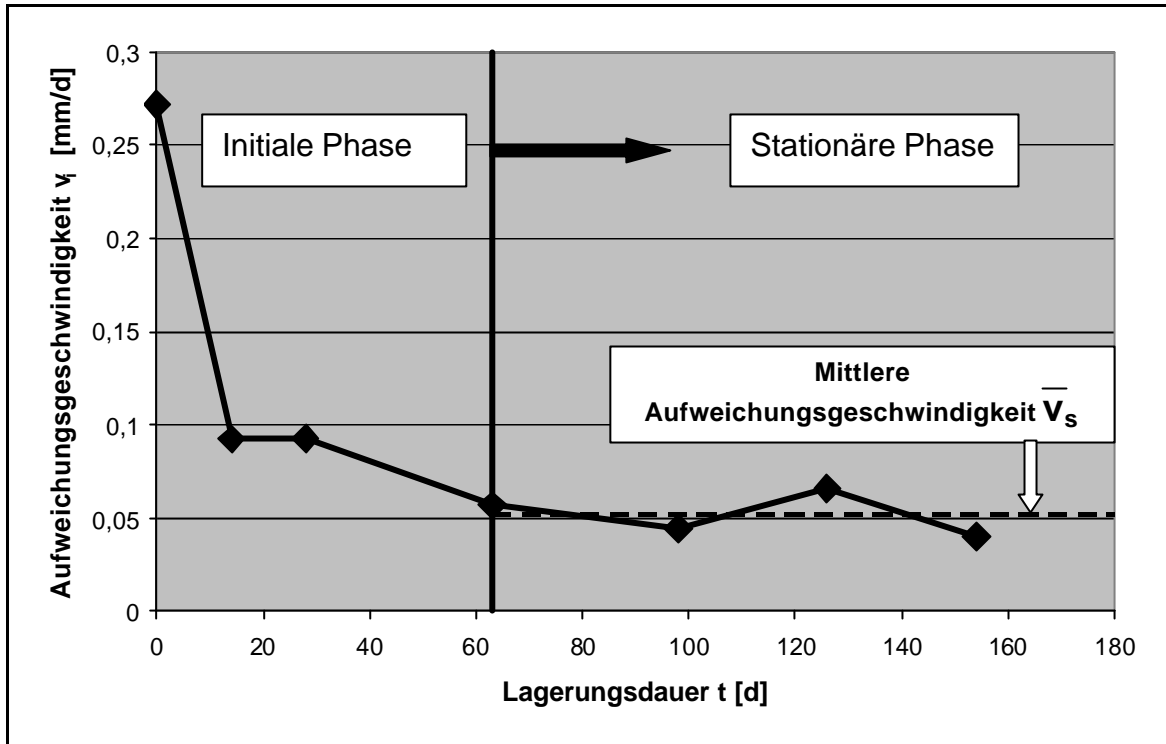
Abb.III.29: Lagerung in kohlenstoffhaltigem Wasser. Aufweichungsgeschwindigkeit v_i als Funktion der Lagerungsdauer t . \text{CO}_{2(\text{aq})} -Konzentration: 100 mg/l. Dichtwand-masse Ca-300.
