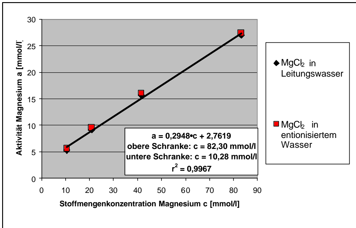
Abb.15: Magnesiumaktivität a einer \text{MgCl}_2 -Lösung als Funktion der Magnesiumkonzentration c. Lösungsmittel Leitungswasser bzw. entionisiertes Wasser.
