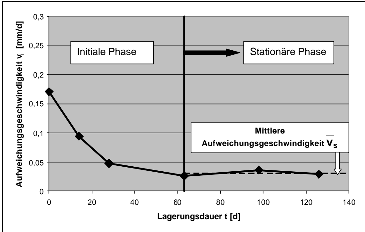
Abb.III.25: Lagerung in kohlensäurehaltigem Wasser. Aufweichungsgeschwindigkeit v_i als Funktion der Lagerungsdauer t . \text{CO}_{2(\text{aq})} -Konzentration: 100 mg/l. Dichtwand-masse: Na-400.
