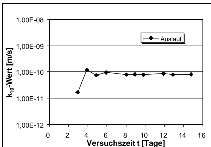
Abb.V.36: Lagerung in Sulfatlösung. k_{10} -Wert in Abhängigkeit von der Versuchsdauer nach 182 Tagen Lagerung. \text{SO}_4^{2-} -Konzentration 15.000 mg/l. Dichtwandmasse Na-230. Messung 3.
