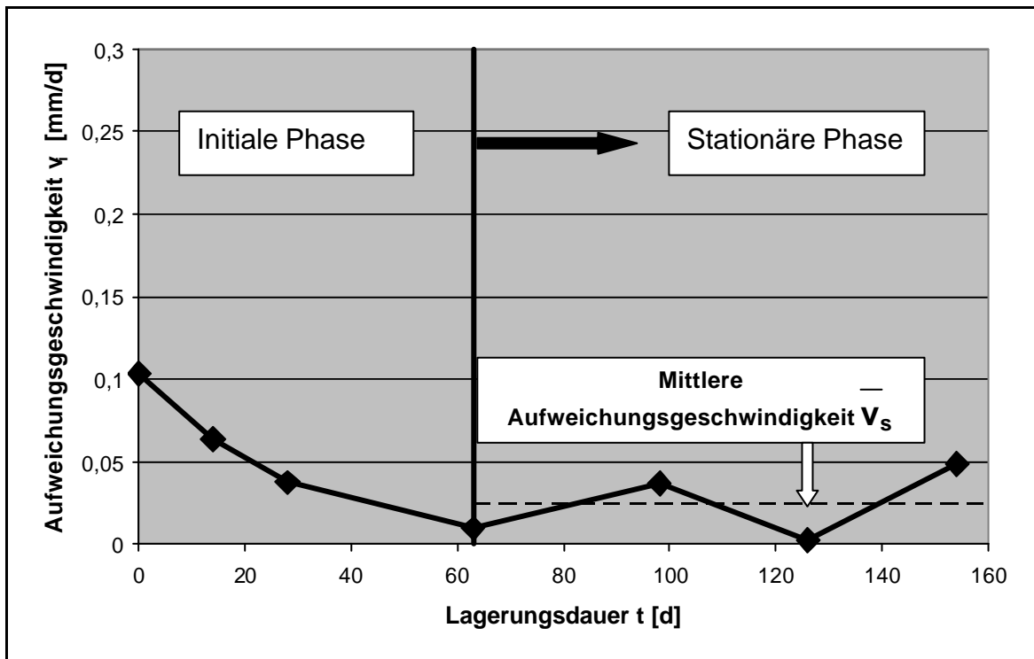
Abb.III.26: Lagerung in kohlensäurehaltigem Wasser. Aufweichungsgeschwindigkeit v_i als Funktion der Lagerungsdauer t . \text{CO}_{2(\text{aq})} -Konzentration: 100 mg/l. Dichtwand-masse Na-540.
