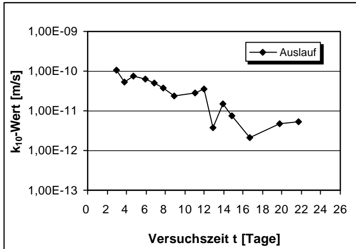
Abb.V.37: Nullprobe. k_{10} -Wert in Abhängigkeit von der Versuchsdauer. Dichtwandmasse Na-540. Messung 2.
