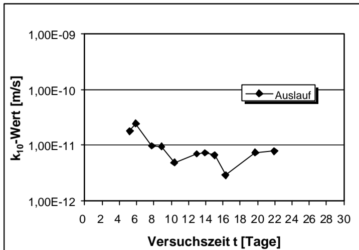
Abb.V.38: Lagerung in Leitungswasser. k_{10} -Wert in Abhängigkeit von der Versuchsdauer nach 28 Tagen Lagerung. Dichtwandmasse Na-540. Messung 1.
