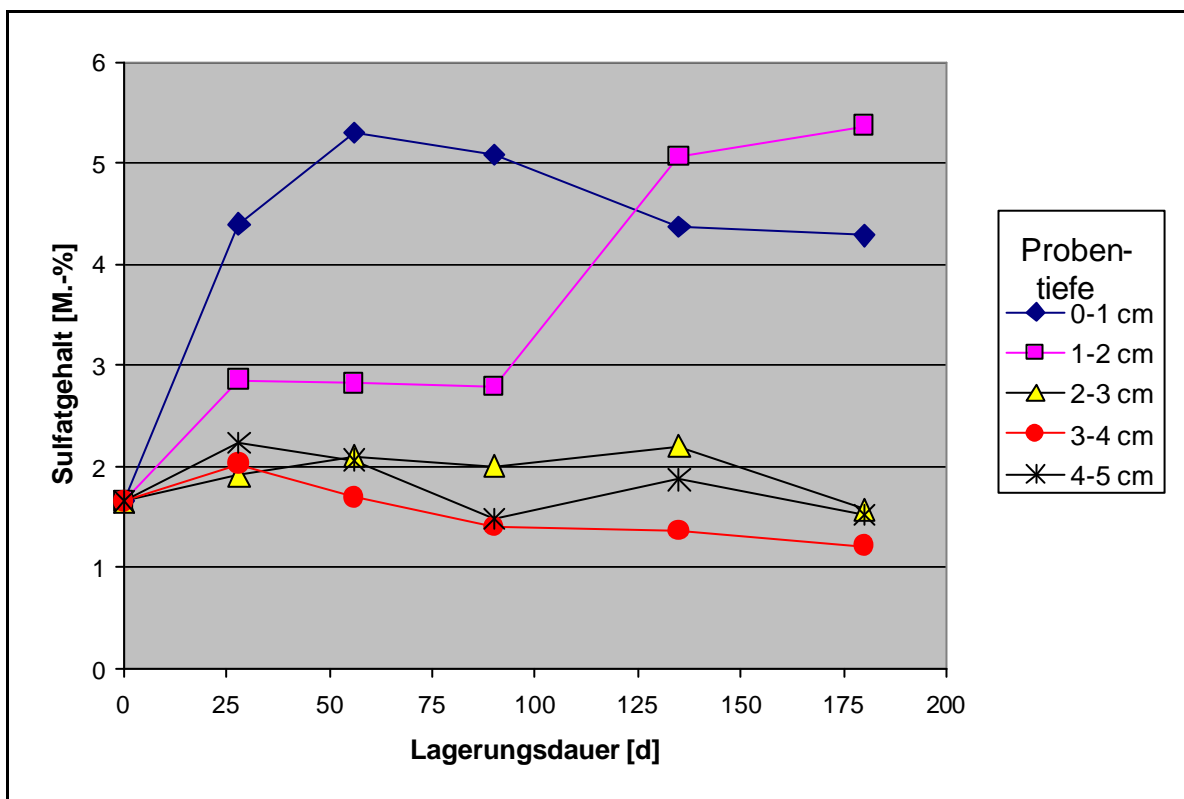
Abb.50: Lagerung in kombinierten Magnesium-/Sulfatlösungen. Sulfatgehalt in Abhängigkeit von der Lagerungsdauer in unterschiedlichen Probertiefen. Mg^{2+} -Konzentration 1.000 mg/l; SO_4^{2-} -Konzentration: 7.500 mg/l. Dichtwandmasse Na -230.
