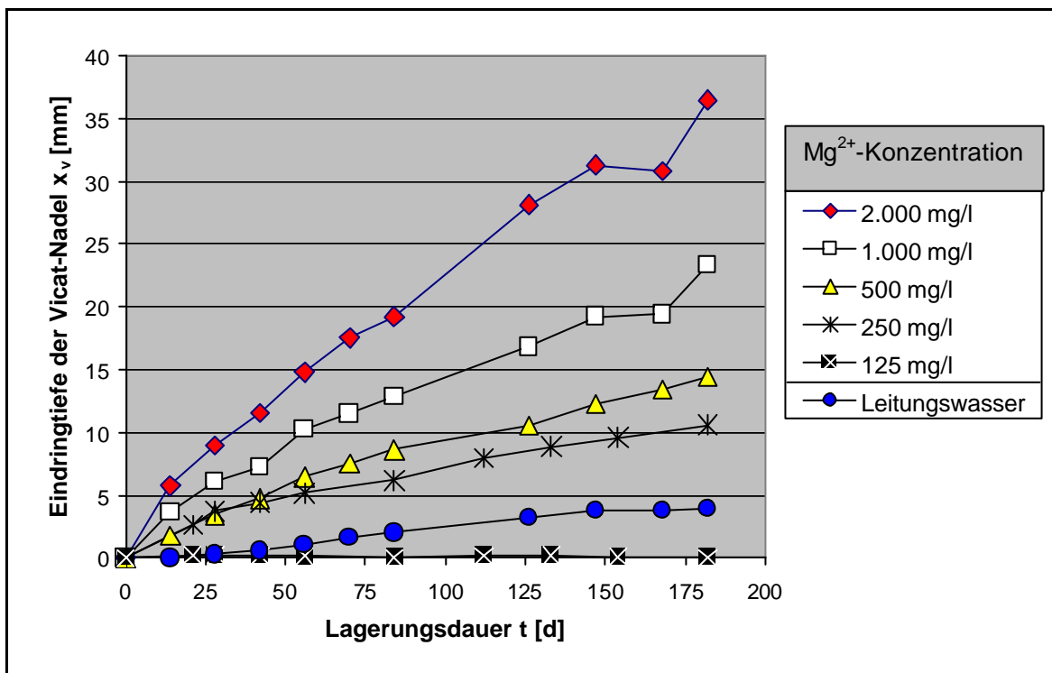
Abb.18: Lagerung in Magnesiumlösungen und Leitungswasser. Eindringtiefe der Vicat-Nadel x_v in Abhängigkeit von der Lagerungsdauer t . Dichtwandmasse Na-230.
