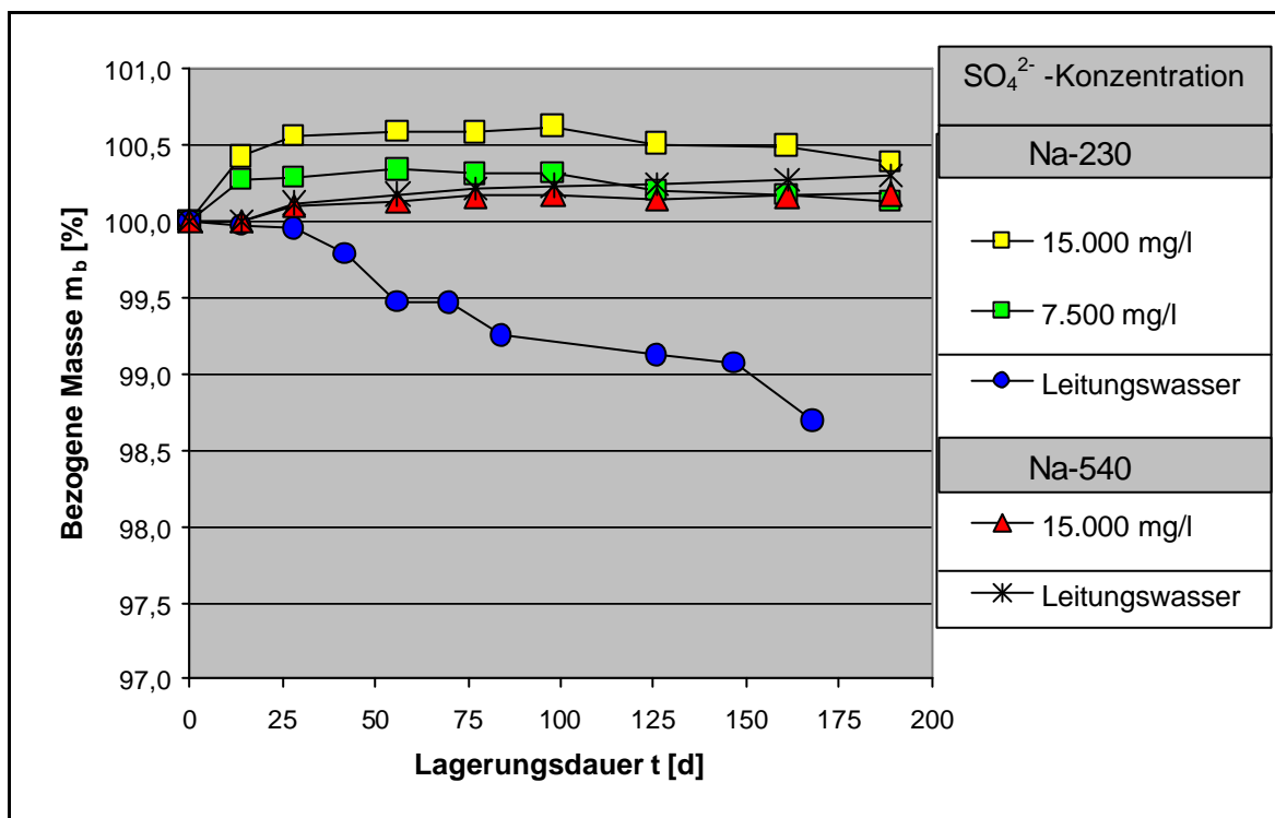
Abb.26: Lagerung in Sulfatlösungen und Leitungswasser. Bezogene Masse m_b in Abhängigkeit von der Lagerungsdauer t. Dichtwandmasse Na-230 und Na-540.
