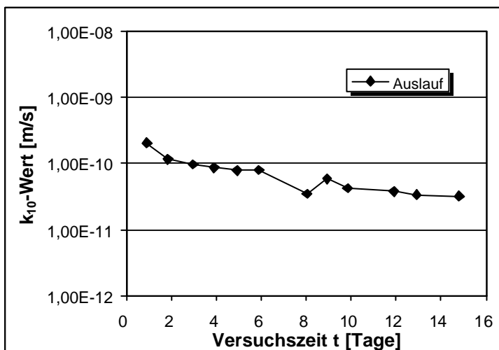
Abb.V.54: Lagerung in Sulfatlösung. k_{10} -Wert in Abhängigkeit von der Versuchsdauer nach 182 Tagen Lagerung. \text{SO}_4^{2-} -Konzentration 15.000 mg/l. Dichtwandmasse Na-540. Messung 1.
