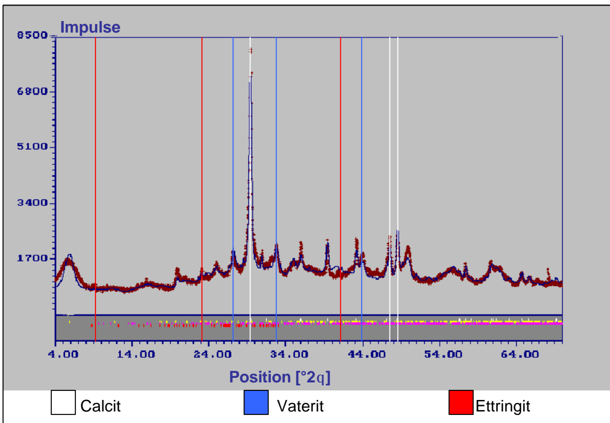
Abb.60: Lagerung in Leitungswasser. Röntgendiffraktogramm der Dichtwandmasse Na-230 nach 182 Tagen. Blaue Kurve: Messwerte. Rote Kurve: Berechnete Werte.
