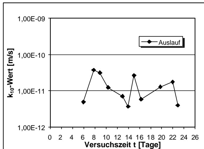
Abb.V.2: Lagerung in Leitungswasser. k_{10} -Wert in Abhängigkeit von der Versuchsdauer nach 28 Tagen Lagerung. Dichtwandmasse Na-230. Messung 1.
