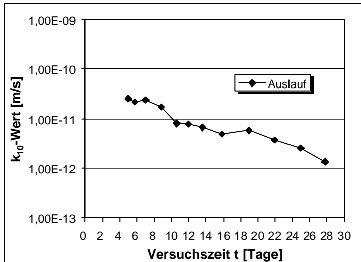
Abb.V.8: Lagerung in Leitungswasser. k_{10} -Wert in Abhängigkeit von der Versuchsdauer nach 98 Tagen Lagerung. Dichtwandmasse Na-230. Messung 1.
