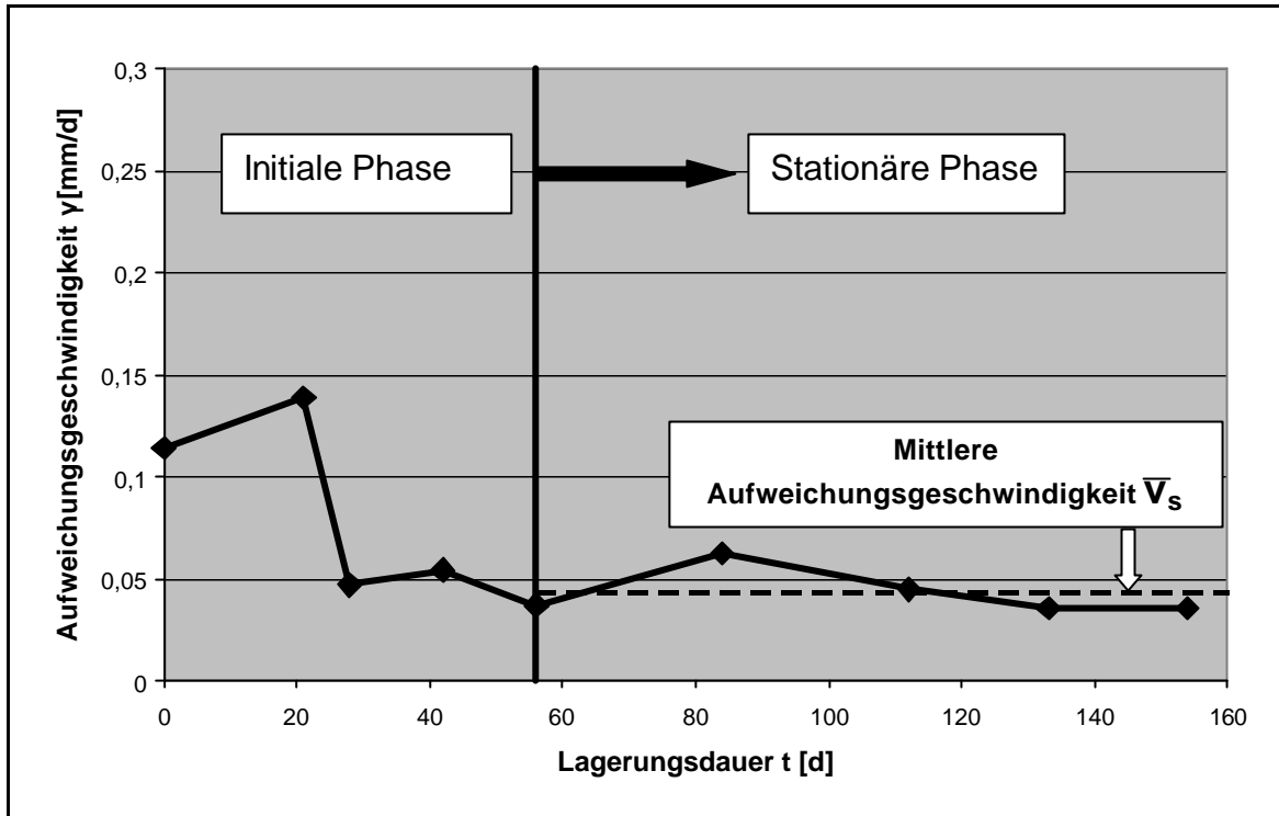
Abb.III.23: Lagerung in Magnesiumlösung. Aufweichungsgeschwindigkeit v_i als Funktion der Lagerungsdauer t . Mg^{2+} -Konzentration: 250 mg/l. Dichtwandmasse Na-230.
