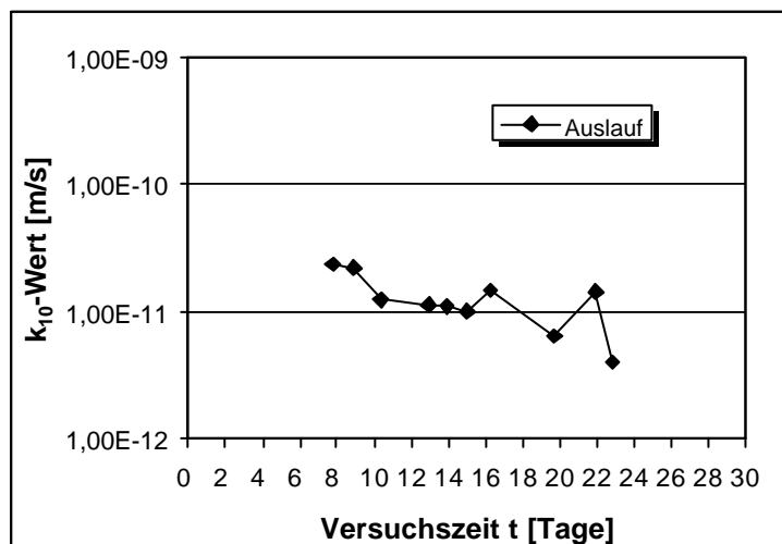
Abb.V.45: Lagerung in Sulfatlösung. k_{10} -Wert in Abhängigkeit von der Versuchsdauer nach 28 Tagen Lagerung. \text{SO}_4^{2-} -Konzentration 15.000 mg/l. Dichtwandmasse Na-540. Messung 2.
