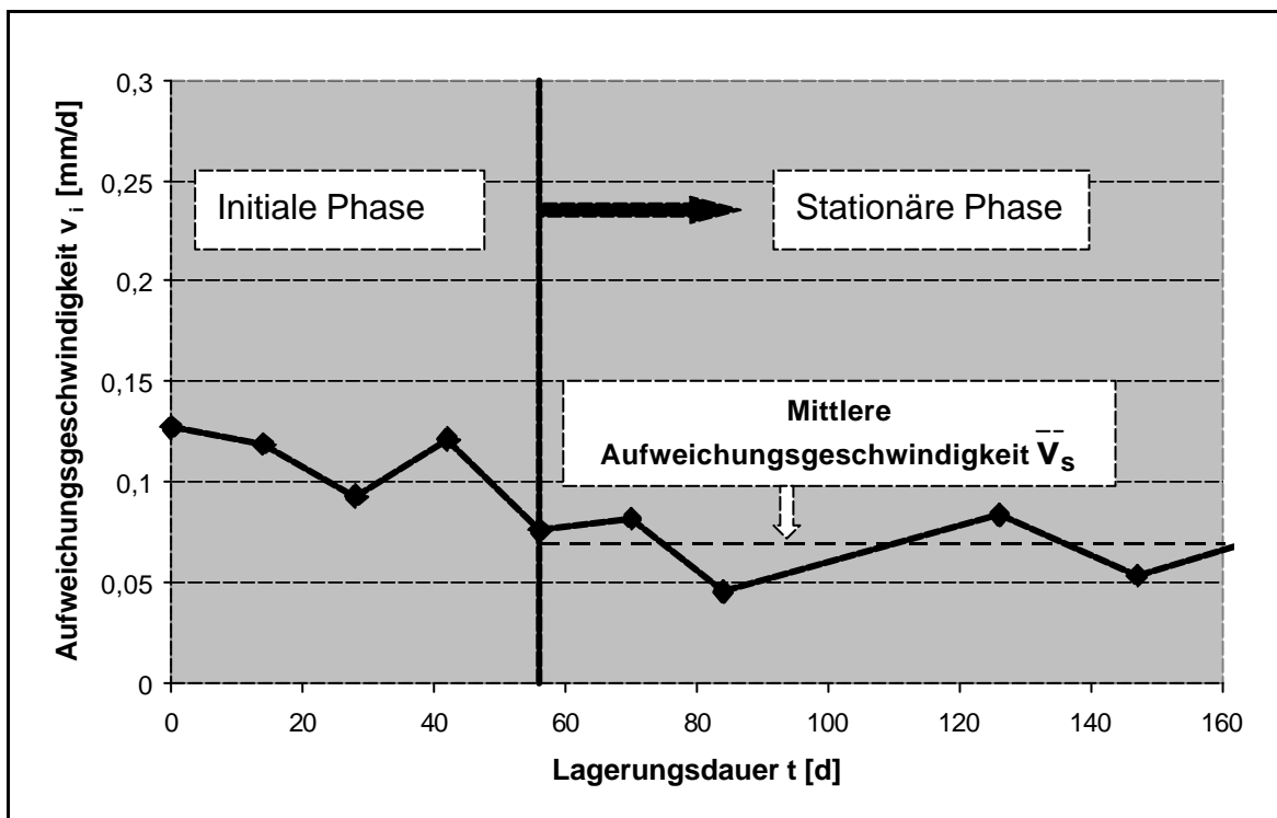
Abb.III.22: Lagerung in Magnesiumlösung. Aufweichungsgeschwindigkeit v_i als Funktion der Lagerungsdauer t . Mg^{2+} -Konzentration: 500 mg/l. Dichtwandmasse Na-230.
