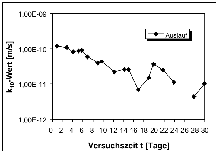
Abb.V.47: Lagerung in Sulfatlösung. k_{10} -Wert in Abhängigkeit von der Versuchsdauer nach 56 Tagen Lagerung. \text{SO}_4^{2-} -Konzentration 15.000 mg/l. Dichtwandmasse Na-540. Messung 2.
