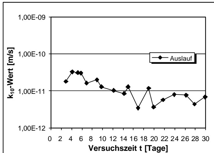
Abb.V.26: Lagerung in Sulfatlösung. k_{10} -Wert in Abhängigkeit von der Versuchsdauer nach 28 Tagen Lagerung. \text{SO}_4^{2-} -Konzentration 15.000 mg/l. Dichtwandmasse Na-230. Messung 4.
