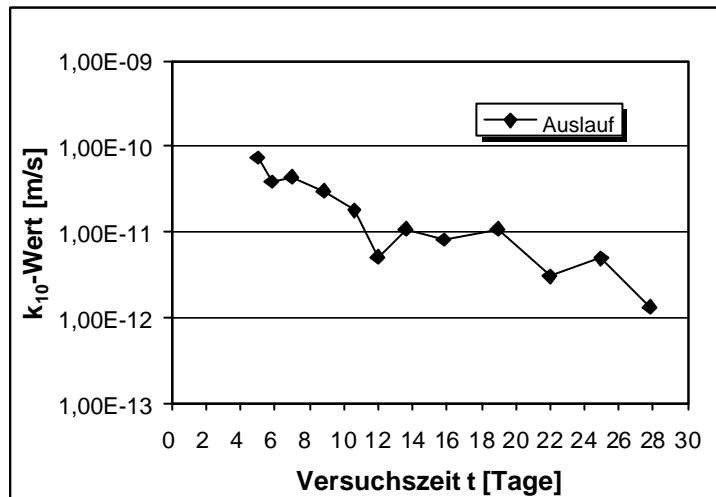
Abb.V.50: Lagerung in Sulfatlösung. k_{10} -Wert in Abhängigkeit von der Versuchsdauer nach 98 Tagen Lagerung. \text{SO}_4^{2-} -Konzentration 15.000 mg/l. Dichtwandmasse Na-540. Messung 1.
