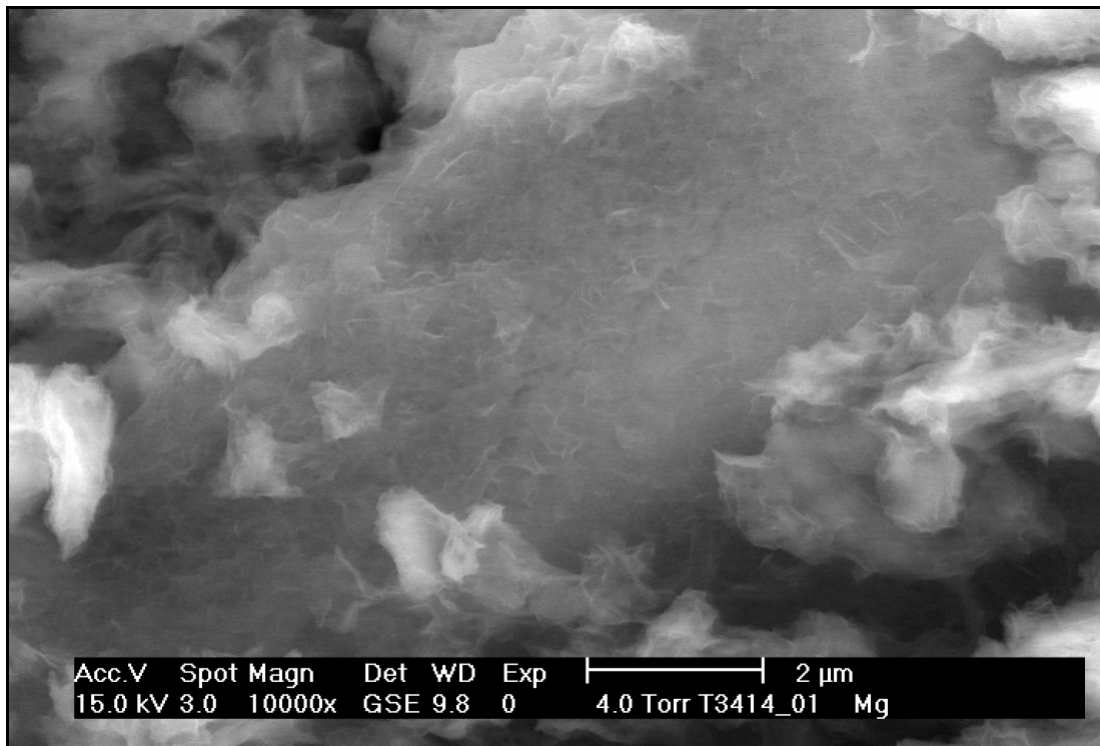
Abb.40: Elektronenmikroskopische Aufnahme (ESEM) der Dichtwandmasse Na-230 nach 182 Tagen Lagerung in Magnesiumlösung ( Mg^{2+} -Konzentration: 2.000 mg/l).
