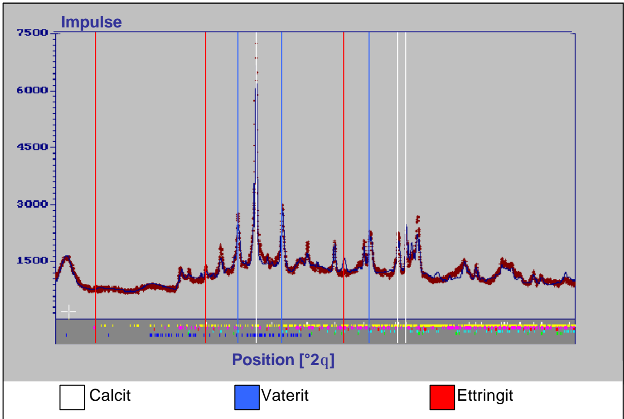
Abb.59: Röntgendiffraktogramm der Nullprobe der Dichtwandmasse Na-230. Blaue Kurve: Messwerte. Rote Kurve: Berechnete Werte.
