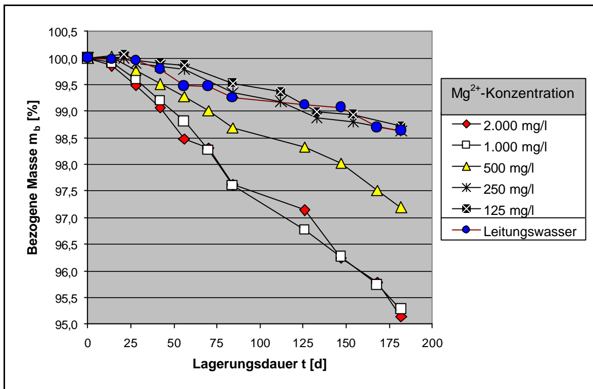
Abb.25: Lagerung in Magnesiumlösungen und Leitungswasser. Bezogene Masse m_b in Abhängigkeit von der Lagerungsdauer t . Dichtwandmasse Na-230.
