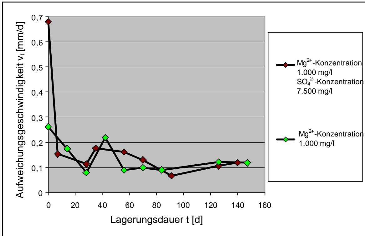
Abb.70: Vergleich Lagerung in Magnesiumlösung mit Lagerung in kombinierter Magnesium-/Sulfatlösung. Aufweichungsgeschwindigkeit v_i in Abhängigkeit von der Lagerungsdauer t . Dichtwandmasse Na-230.
