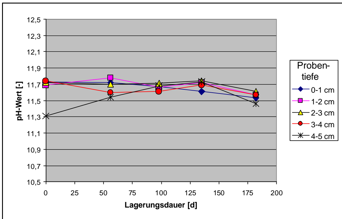
Abb.53: Lagerung in Leitungswasser. pH-Wert der Dichtwandmasse Na-230 in Abhängigkeit von der Lagerungsdauer in unterschiedlichen Probertiefen.
