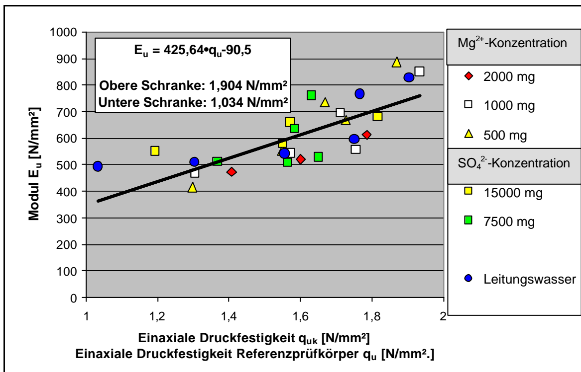
Abb.32: Lagerung in Magnesiumlösungen, Sulfatlösungen und Leitungswasser. Modul des einaxialen Druckversuches E_u als Funktion der einaxialen Druckfestigkeit der in Schadstofflösung gelagerten Prüfkörper q_{uk} und der Referenzprüfkörper q_u . Dichtwandmasse Na-230.
