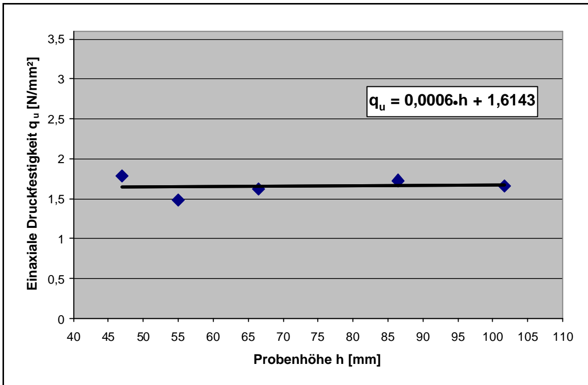
Abb.IV.1: Vorversuche. Einaxiale Druckfestigkeit q_u als Funktion der Probenhöhe h bei einem h/d -Verhältnis von 1. Dichtwandmasse Na-230. Probenalter 56 Tage.
