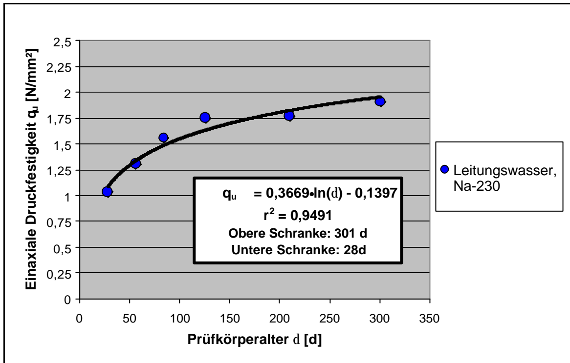
Abb.29: Lagerung in Leitungswasser. Einaxiale Druckfestigkeit q_u als Funktion des Prüfkörperalters \delta . Dichtwandmasse Na-230.
