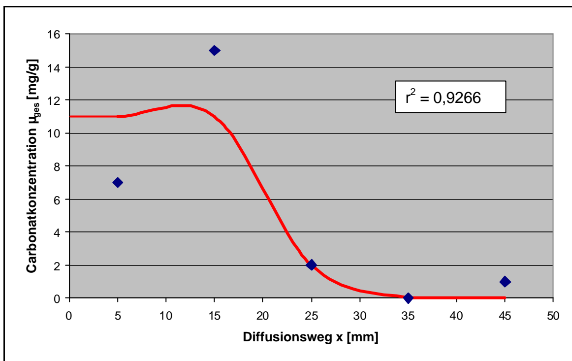
Abb.72: Lagerung in kohlensäurehaltigem Wasser. Carbonatkonzentration \mu_{\text{ges}} in Abhängigkeit vom Diffusionsweg x nach 182 Tagen Lagerungsdauer. \text{CO}_{2(\text{aq})}^- Konzentration: 100 mg/l. Dichtwandmasse Na-230. Blau: Messwerte. Rot: iterativ berechnetes Diffusionsprofil.
