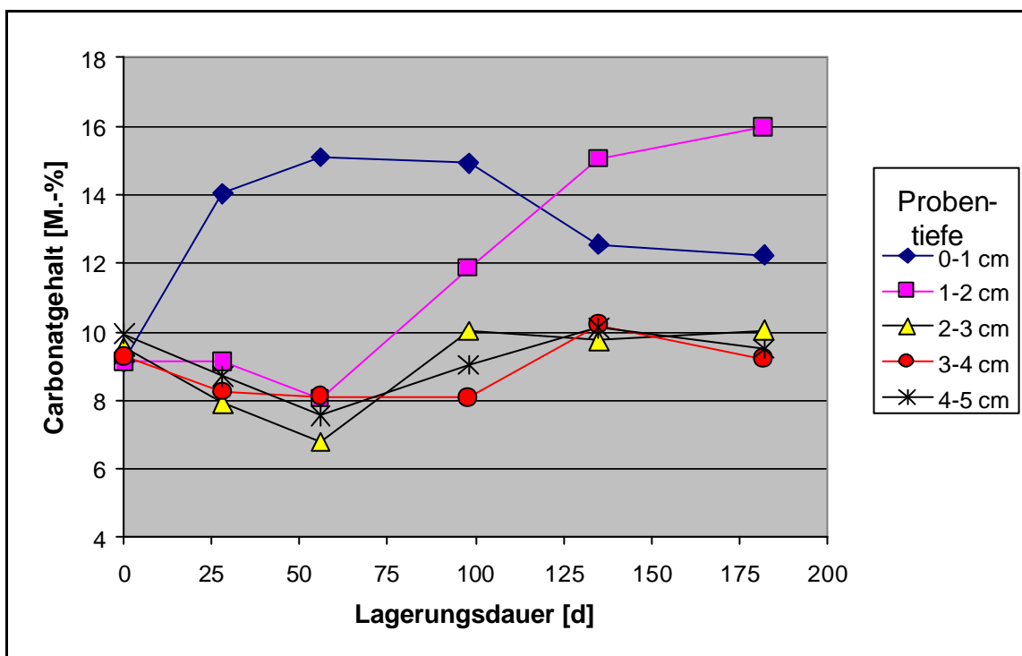
Abb.58: Lagerung in kohlensäurehaltigem Wasser. Carbonatgehalt in Abhängigkeit von der Lagerungsdauer in unterschiedlichen Probentiefen. \text{CO}_{2(\text{aq})} -Konzentration: 100 mg/l. Dichtwandmasse Na-230.
