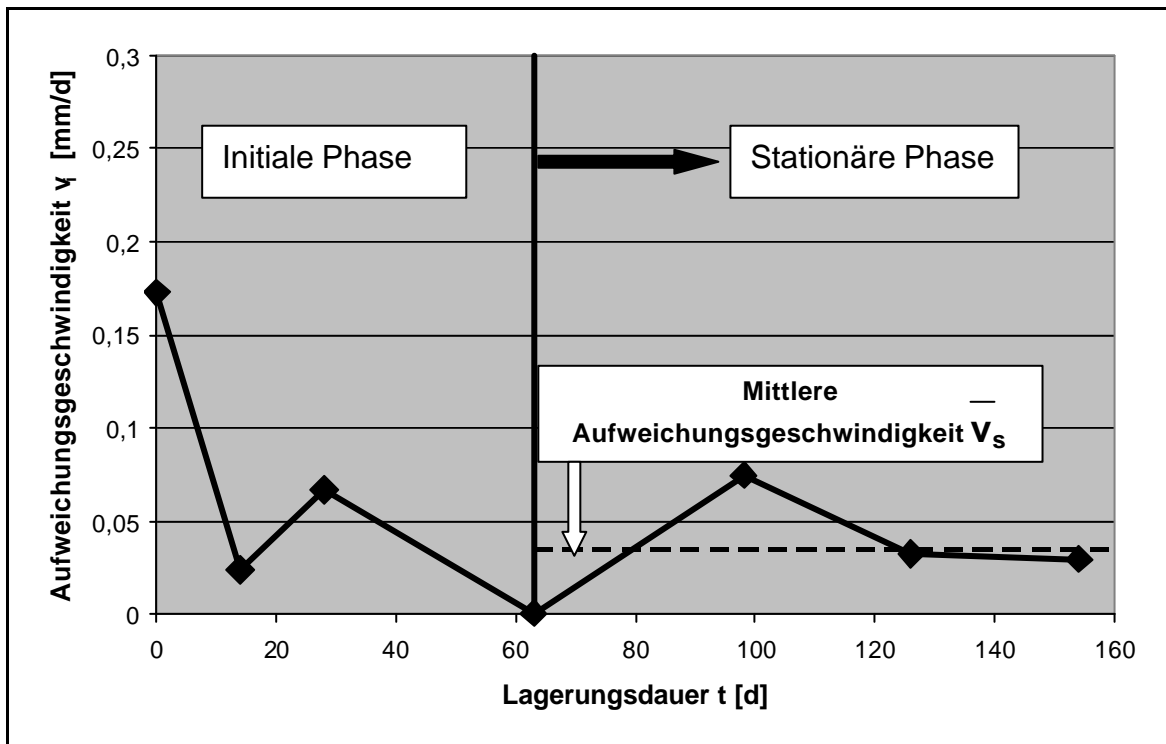
Abb.III.30: Lagerung in kohlenstoffhaltigem Wasser. Aufweichungsgeschwindigkeit v_i als Funktion der Lagerungsdauer t . \text{CO}_{2(\text{aq})} -Konzentration: 100 mg/l. Dichtwand-masse Ca-400.
