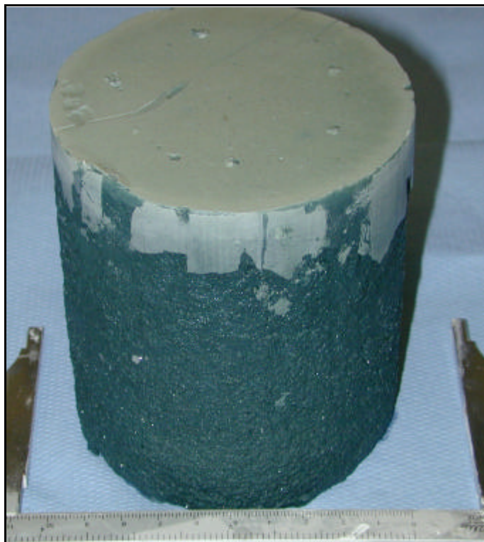
Abb.II.2: Lagerung in einer kombinierten Magnesium-/Sulfatlösung. Prüfkörper der Dichtwandmasse Na-230 mit beginnenden Ablösungserscheinungen im oberflächennahen Bereich nach 28 Tagen Lagerungsdauer. Mg^{2+} -Konzentration: 1.000 mg/l; SO_4^{2-} -Konzentration: 7.500 mg/l.
