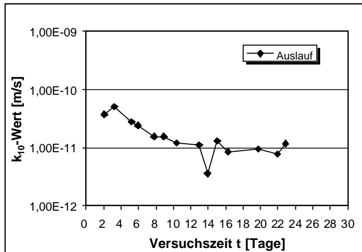
Abb.V.44: Lagerung in Sulfatlösung. k_{10} -Wert in Abhängigkeit von der Versuchsdauer nach 28 Tagen Lagerung. \text{SO}_4^{2-} -Konzentration 15.000 mg/l. Dichtwandmasse Na-540. Messung 1.
