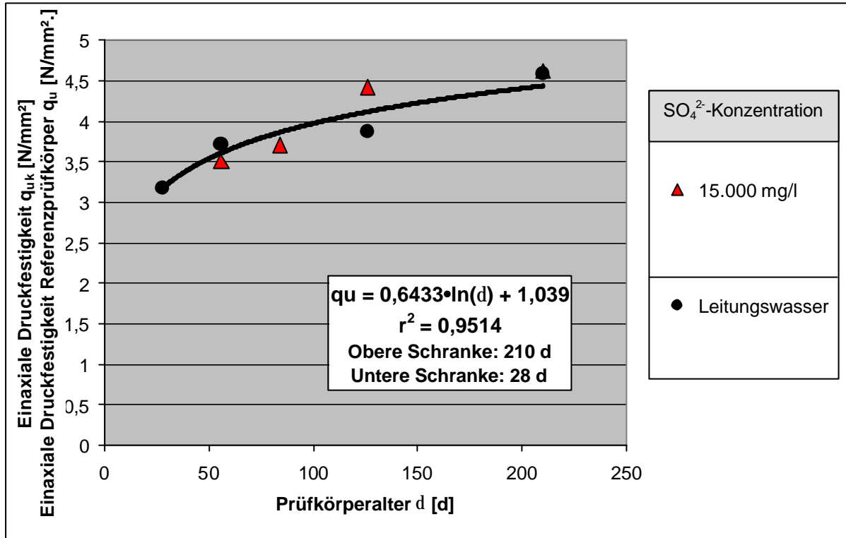
Abb.34: Lagerung in Sulfatlösung und Leitungswasser. Einaxiale Druckfestigkeit der in Sulfatlösung gelagerten Prüfkörper q_{uk} und der Referenzprüfkörper q_u als Funktion des Prüfkörperalters \delta . Dichtwandmasse Na-540.
