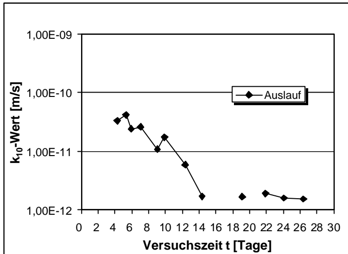
Abb.V.7: Lagerung in Leitungswasser. k_{10} -Wert in Abhängigkeit von der Versuchsdauer nach 56 Tagen Lagerung. Dichtwandmasse Na-230. Messung 3.
