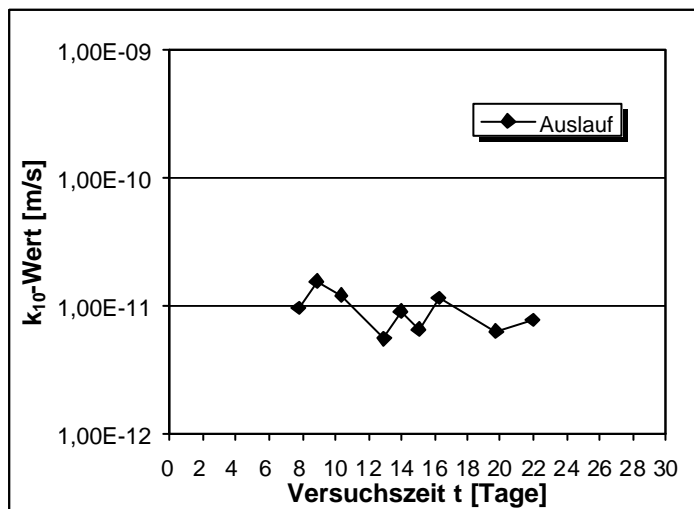
Abb.V.3: Lagerung in Leitungswasser. k_{10} -Wert in Abhängigkeit von der Versuchsdauer nach 28 Tagen Lagerung. Dichtwandmasse Na-230. Messung 2.
