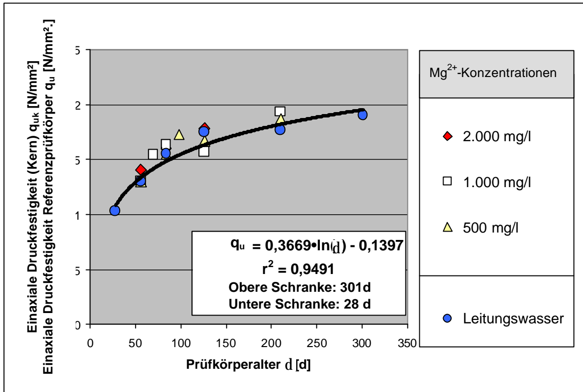
Abb.30: Lagerung in Magnesiumlösungen und Leitungswasser. Einaxiale Druckfestigkeit des Prüfkörperkerns q_{uk} und einaxiale Druckfestigkeit der Referenzprüfkörper q_u als Funktion des Prüfkörperalters \delta . Dichtwandmasse Na-230.
