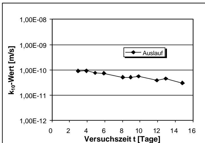
Abb.V.21: Lagerung in Sulfatlösung. k_{10} -Wert in Abhängigkeit von der Versuchsdauer nach 182 Tagen Lagerung. \text{SO}_4^{2-} -Konzentration 7.500 mg/l. Dichtwandmasse Na-230. Messung 3.
