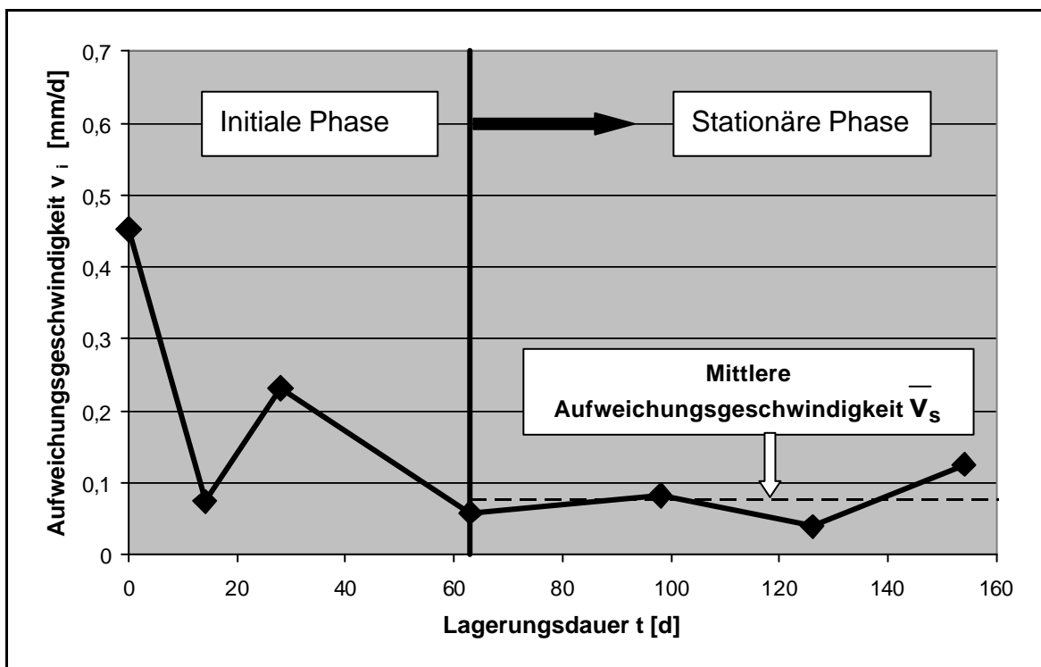
Abb.III.28: Lagerung in kohlenensäurehaltigem Wasser. Aufweichungsgeschwindigkeit v_i als Funktion der Lagerungsdauer t . \text{CO}_{2(\text{aq})} -Konzentration: 100 mg/l. Dichtwand-masse Na-250KK.
