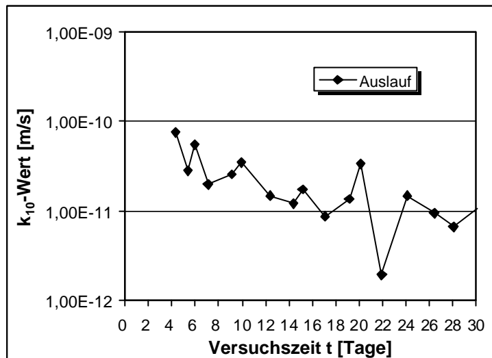
Abb.V.5: Lagerung in Leitungswasser. k_{10} -Wert in Abhängigkeit von der Versuchsdauer nach 56 Tagen Lagerung. Dichtwandmasse Na-230. Messung 1.
