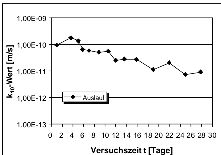
Abb.V.51: Lagerung in Sulfatlösung. k_{10} -Wert in Abhängigkeit von der Versuchsdauer nach 98 Tagen Lagerung. \text{SO}_4^{2-} -Konzentration 15.000 mg/l. Dichtwandmasse Na-540. Messung 2.
