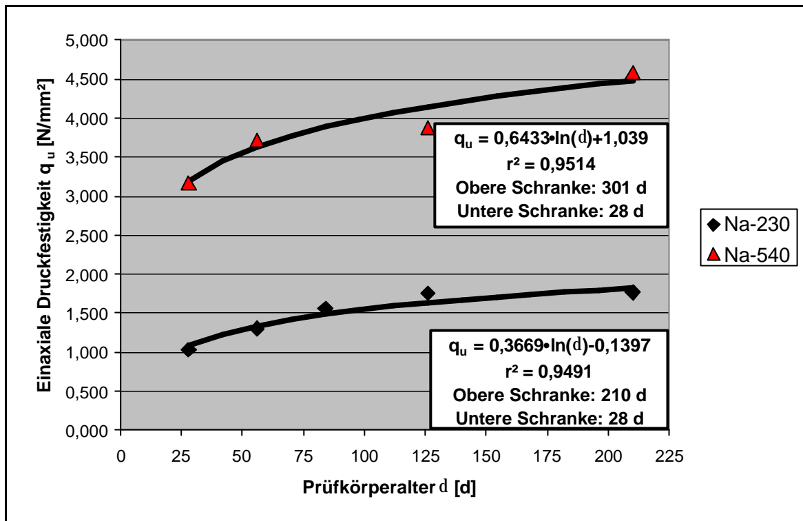
Abb.66: Lagerung in Leitungswasser. Einaxiale Druckfestigkeit q_u der Dichtwandmassen Na-230 und Na-540 in Abhängigkeit vom Prüfkörperalter \delta .
