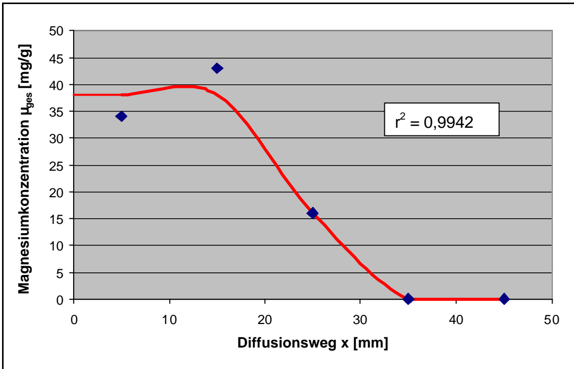
Abb.68: Lagerung in Magnesiumlösung. Magnesiumkonzentration \mu_{ges} in Abhängigkeit vom Diffusionsweg x nach 182 Tagen Lagerungsdauer. Mg^{2+} -Konzentration 2.000 mg/l. Dichtwandmasse Na-230. Blau: Messwerte. Rot: iterativ berechnetes Diffusionsprofil.
