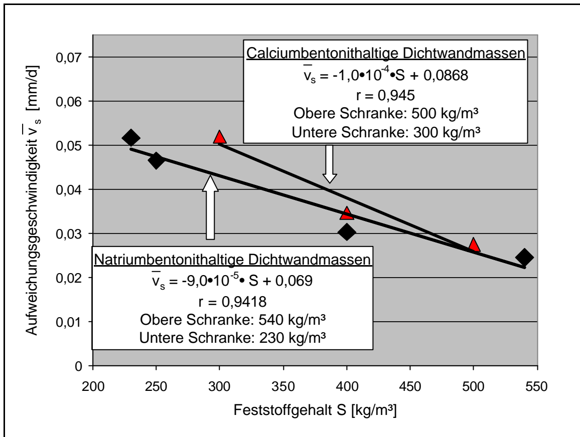
Abb. 73: Lagerung in kohlensäurehaltigem Wasser. Aufweichungsgeschwindigkeit in der stationären Phase \bar{v}_s als Funktion des Feststoffgehaltes S. \text{CO}_{2(\text{aq})} -Konzentration: 100 mg/l. Natriumbentonithaltige Dichtwandmassen (Na-230, Na-250, Na-400, Na-540); calciumbentonithaltige Dichtwandmassen (Ca-300, Ca-400, Ca-500).
