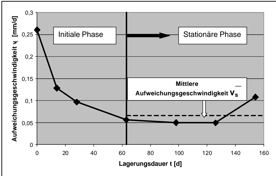
Abb.III.27: Lagerung in kohlenensäurehaltigem Wasser. Aufweichungsgeschwindigkeit v_i als Funktion der Lagerungsdauer t . \text{CO}_{2(\text{aq})} -Konzentration: 100 mg/l. Dichtwand-masse Na-250K.
