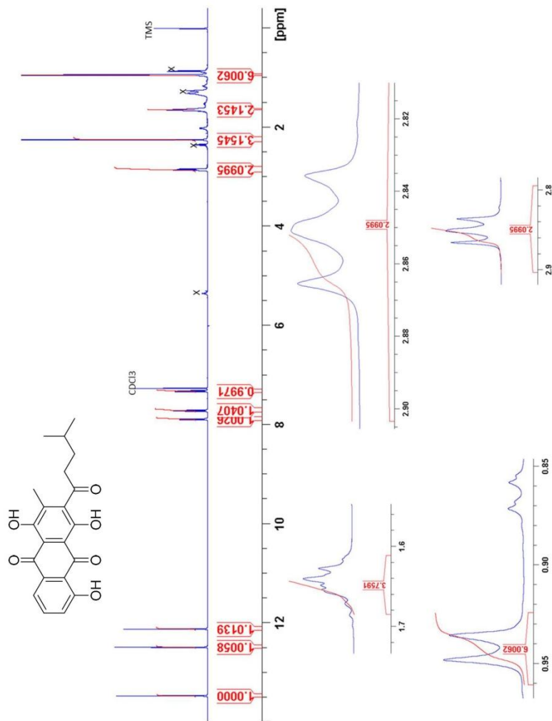
Suppl. Fig. 16. 1 H Galvaquinone B (2).
