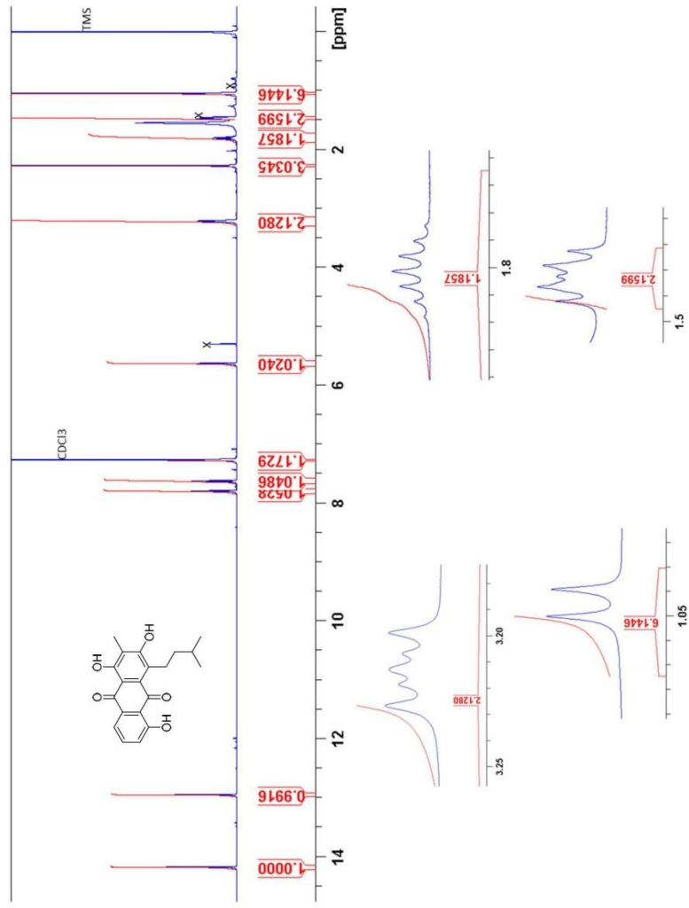
Suppl. Fig. 11. 1 H NMR of Lupinacinin A (1).
