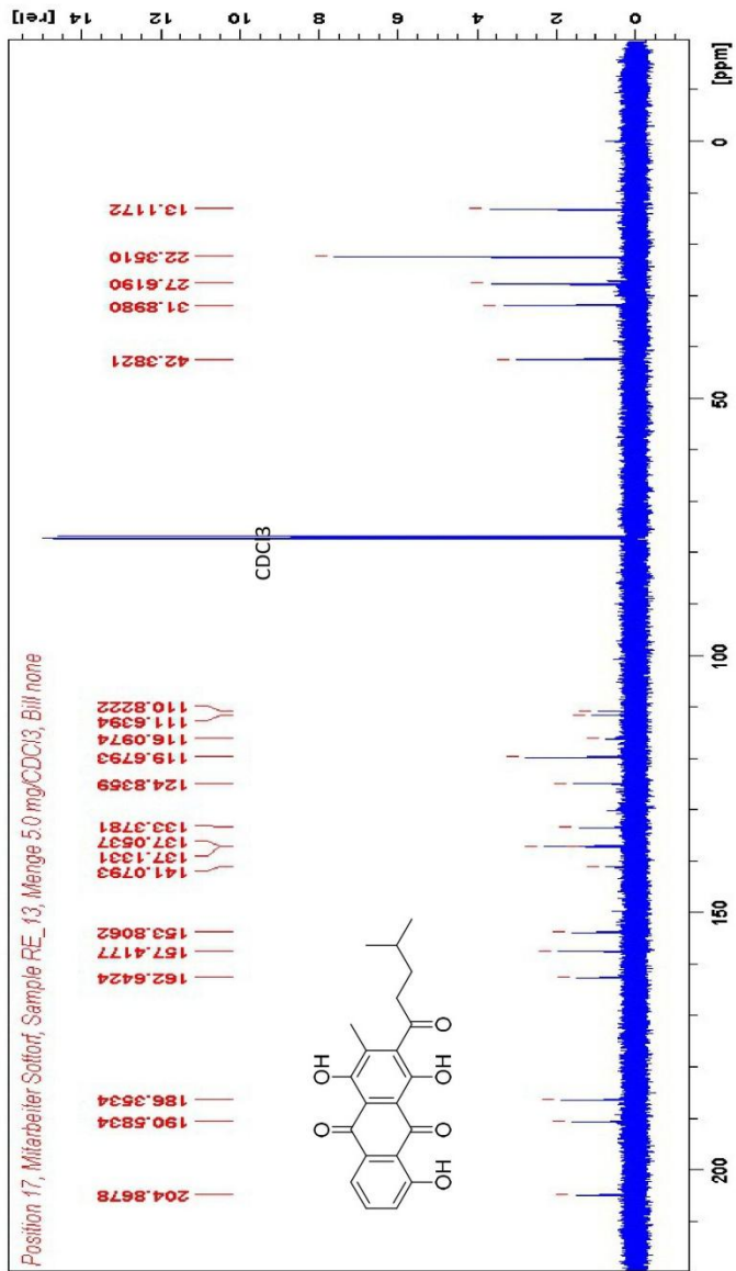
Suppl. Fig. 17. 13 C Galvaquinone B (2).
