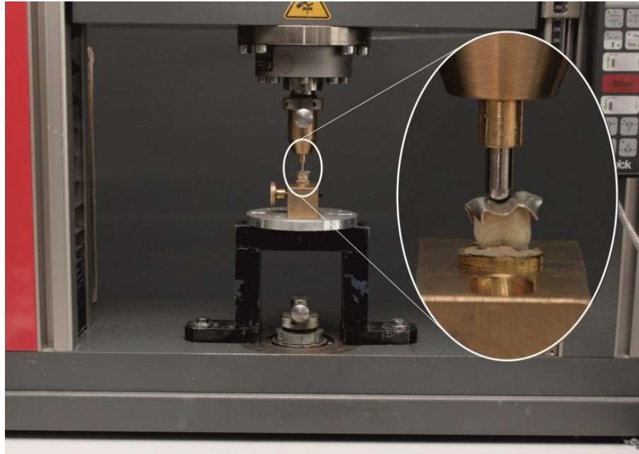
Fig. 19. Universal testing machine (Zwick Z010/TN2A)
